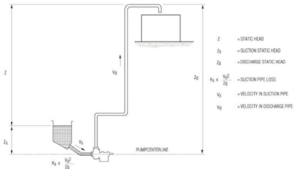
شکل ۳-۷: کاربرد نمونه ای پمپ
