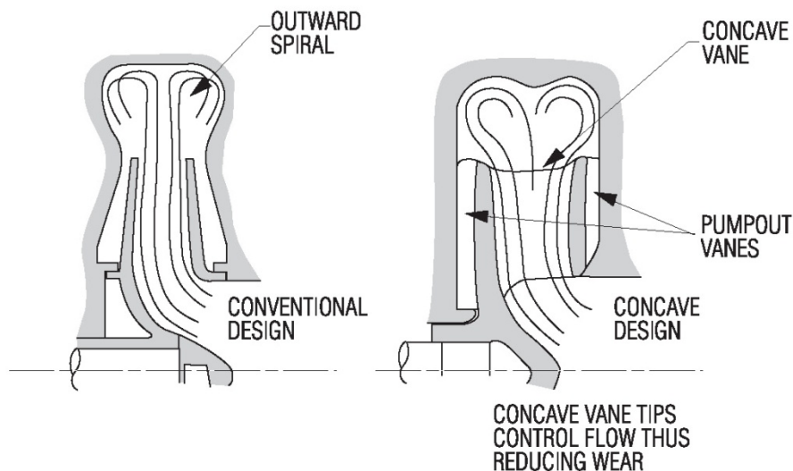
شکل ۳-۱: الگوهای جریان پروانه/پوسته
