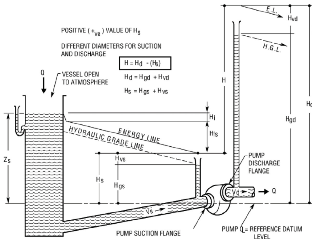
شکل ۳-۵: هد دینامیکی کلی با هد ورودی مثبت
