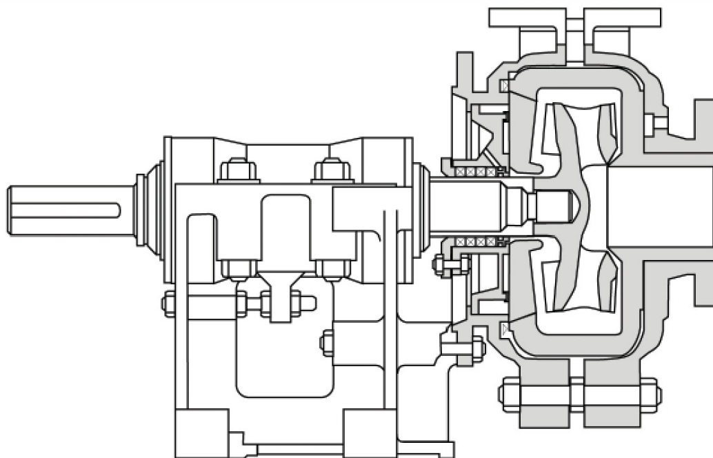
شکل ۴-۱: پمپ OH1/SL
