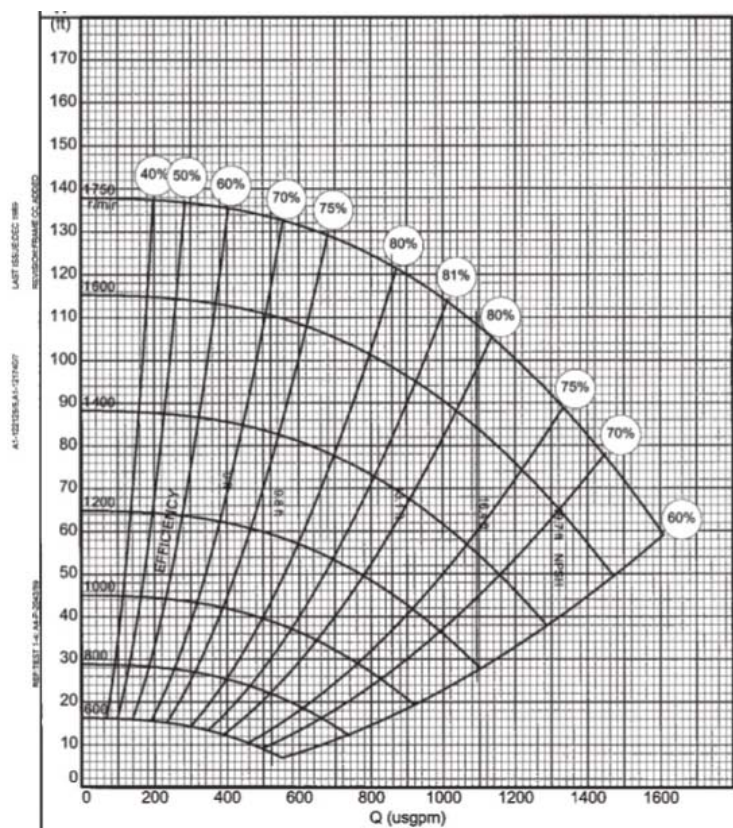
شکل ۳-۸: منحنی عملکرد پمپ
