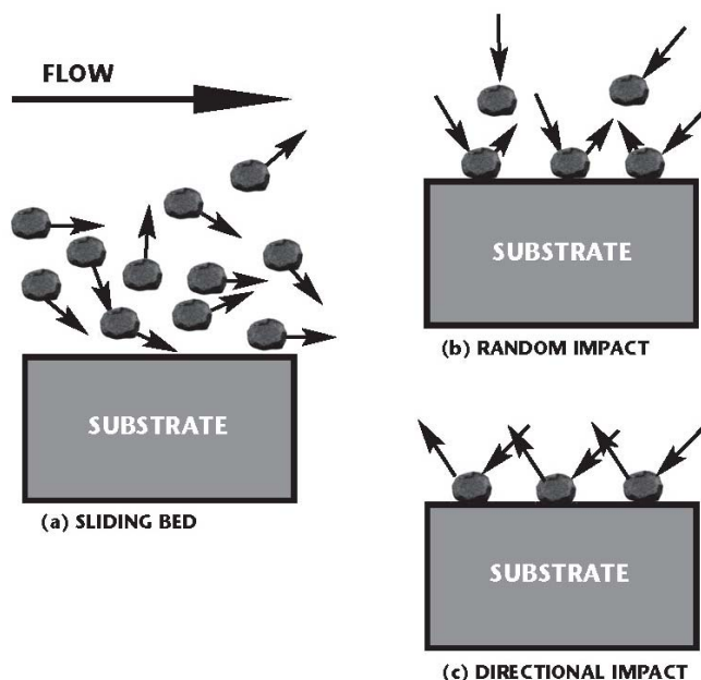
شکل ۲-۲: سه نوع اصلی سایش Erosion
