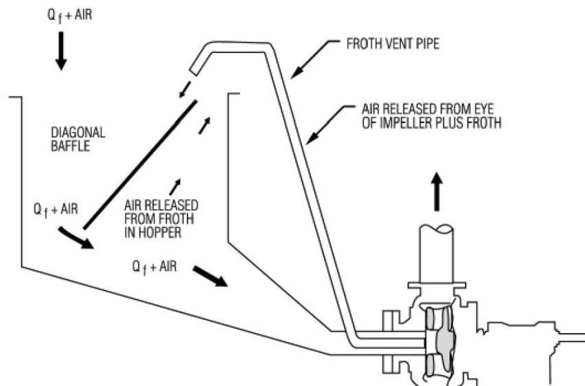
شکل ۲-۱۰: یک نمونه از جانمایی مخزن پمپ برای اسلاری های کف آلود و اسفنجی
