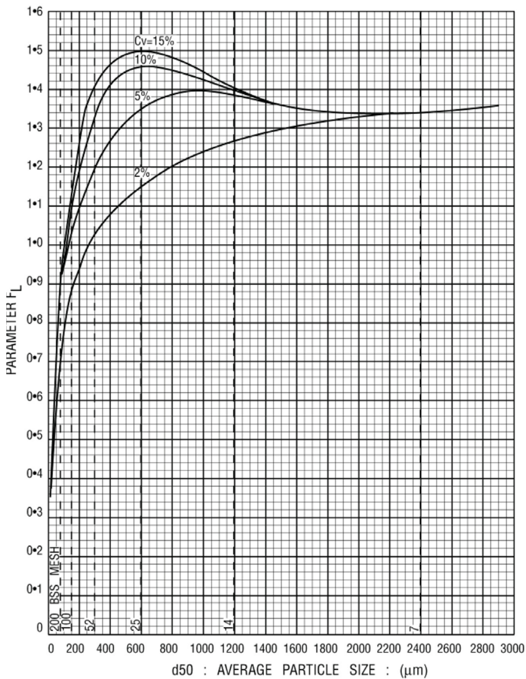
شکل ۷-۱: نمودار F_L برای ذرات بصورت نزدیک دانه بندی شده - معادله دوران
