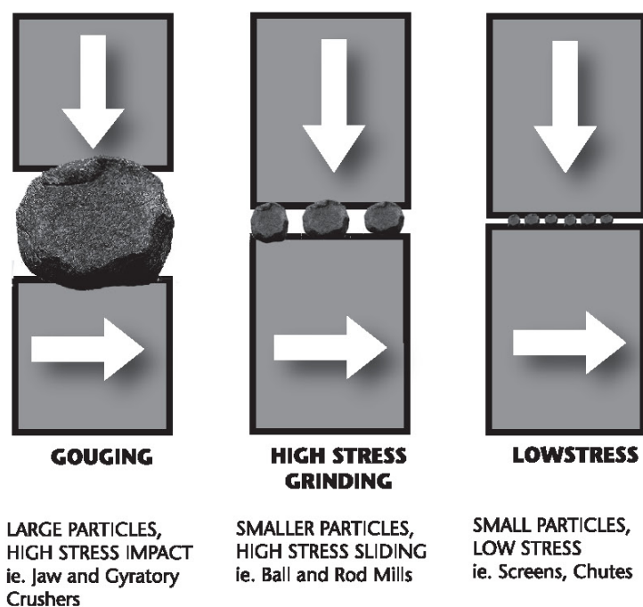
شکل ۱-۲: سه نوع اصلی سایش Abrasion
