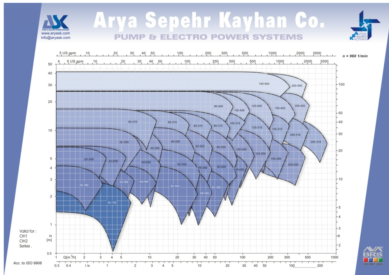
شکل ۱-۳: منحنی همپوشانی پمپ سانتریفوژ اسلاری مدل OH1/SL
