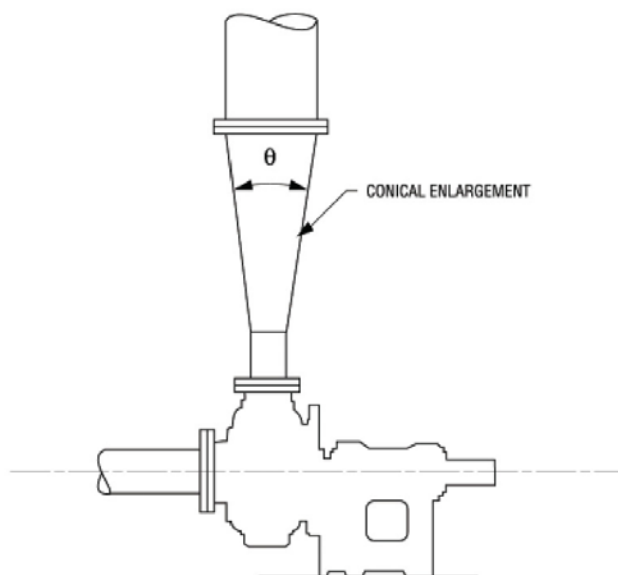
شکل ۳-۲: تبدیل انبساطی مخروطی
