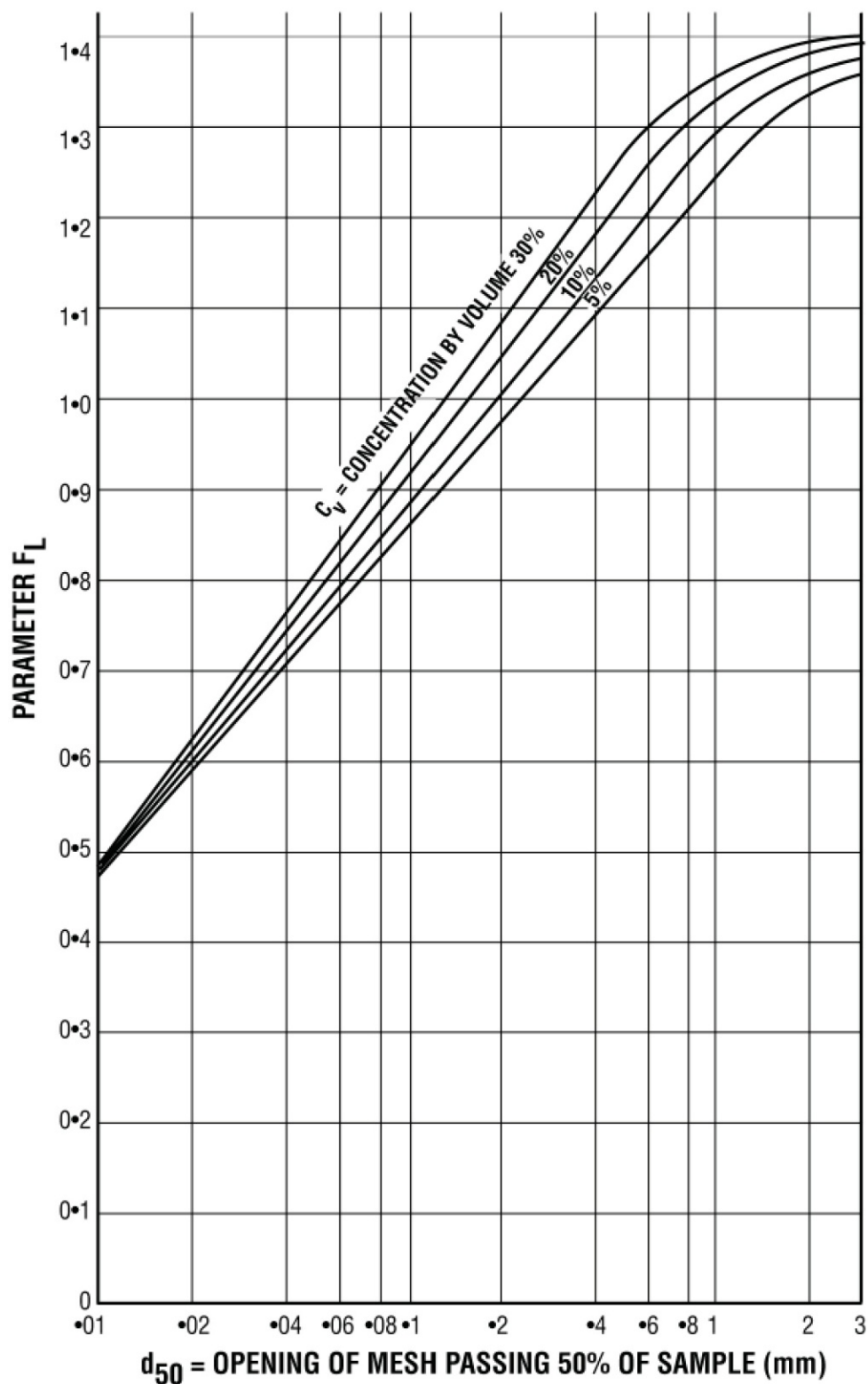
شکل ۷-۲: نمودار F_L برای ذرات بصورت گسترده دانه بندی شده - معادله دوراند
