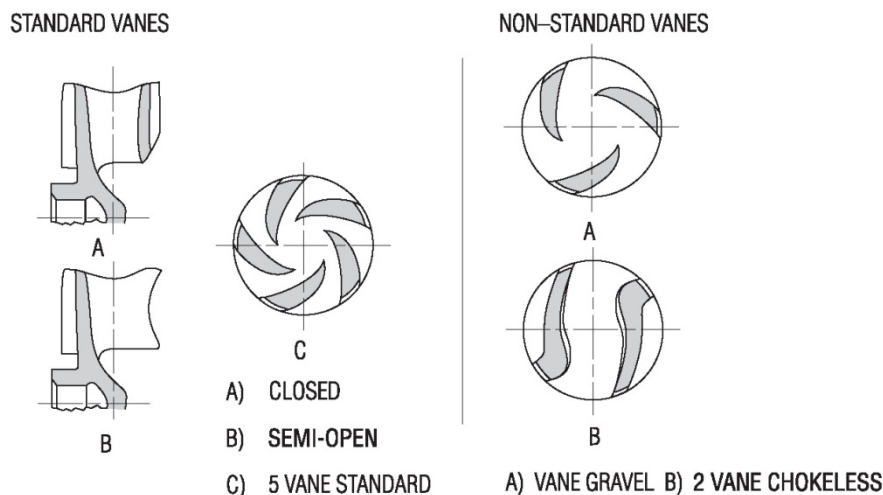
شکل ۳-۱: انواع پروانه استاندارد و غیر استاندارد (ویژه)
