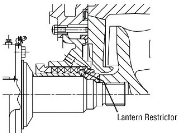
شکل ۲-۸: نمای آببند نوار گرافیتی (گلند پکینگ)
