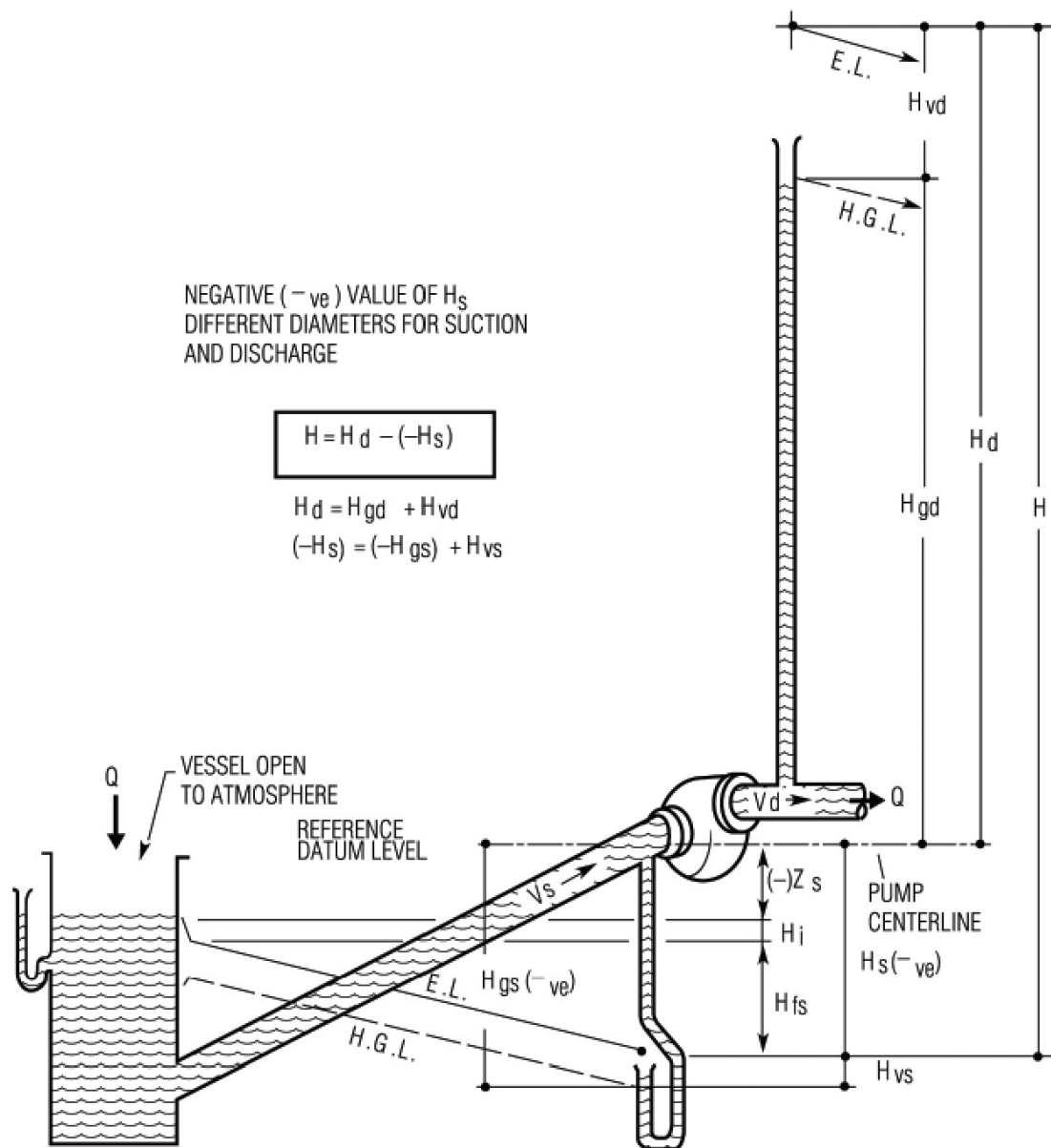
شکل ۳-۶: هد دینامیکی کلی با هد ورودی منفی
