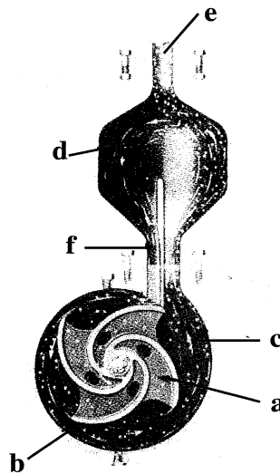
شکل ۵ پمپ خودمکش با بازچرخش در رانش
